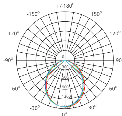
35W 4000K
