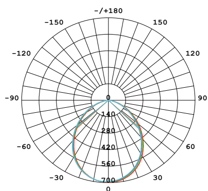
18W 4000K
